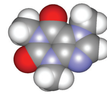
Struktur von Koffein
