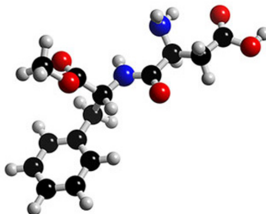
Dreidimensionale Struktur von Aspartam (mit dem Link gelangt man zu einer Website, auf der das Molekül drehbar ist:
